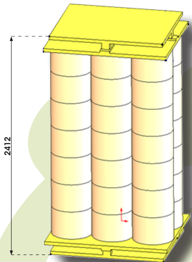
DIMENSIONES APROX. PALETIZADO TIPO EURO O SIMILAR
